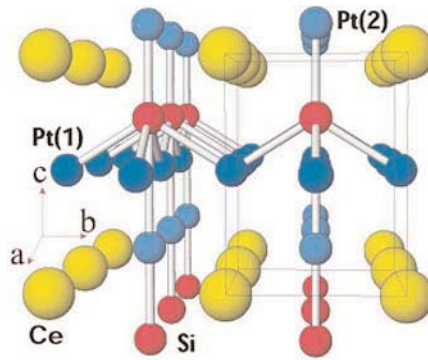
Abb. 1: Kristallstruktur von CePt_3Si . Die Struktur ist tetragonal, zeigt aber in Richtung der polaren c-Achse kein symmetrisches Verhalten (= Fehlen eines Inversionszentrums)
