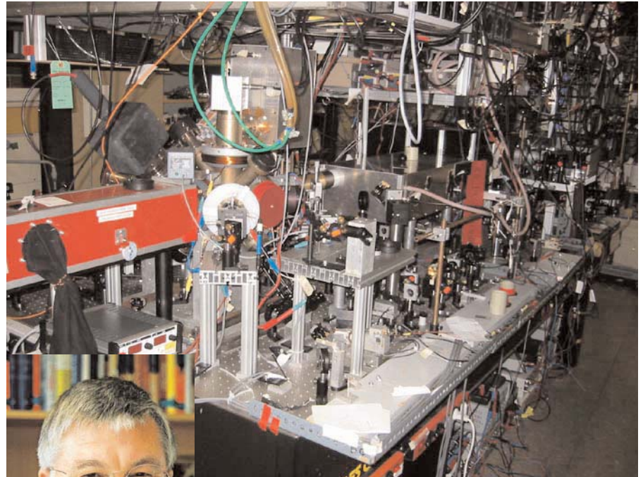
Versuchsanordnung in der Universität Innsbruck
